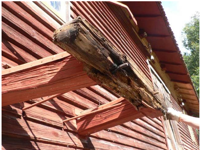
Rötskadade delar på stöd för drivhjul till spånhyvel mm på sågens utsida.
